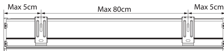
Innenhalterung
